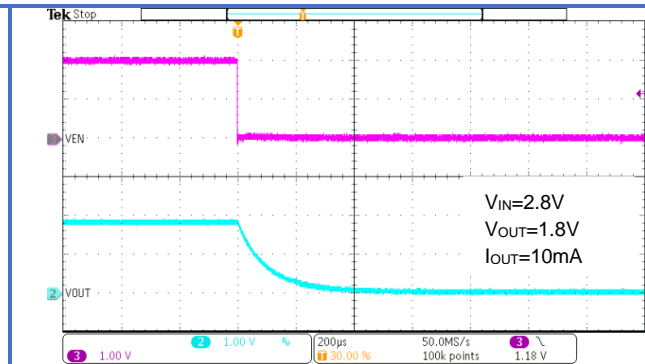
Figure 29. EN Shutdown
